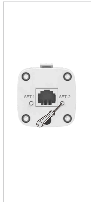
3. 电机通电, 长按【SET-2】键至指示灯闪烁
